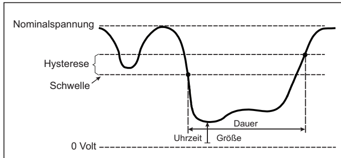
Abbildung 13. Merkmale einer Spannungsunterbrechung
