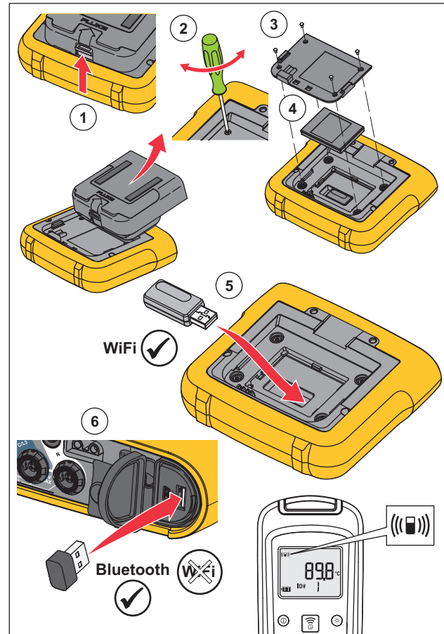
Abbildung 1. Adapterinstallation
