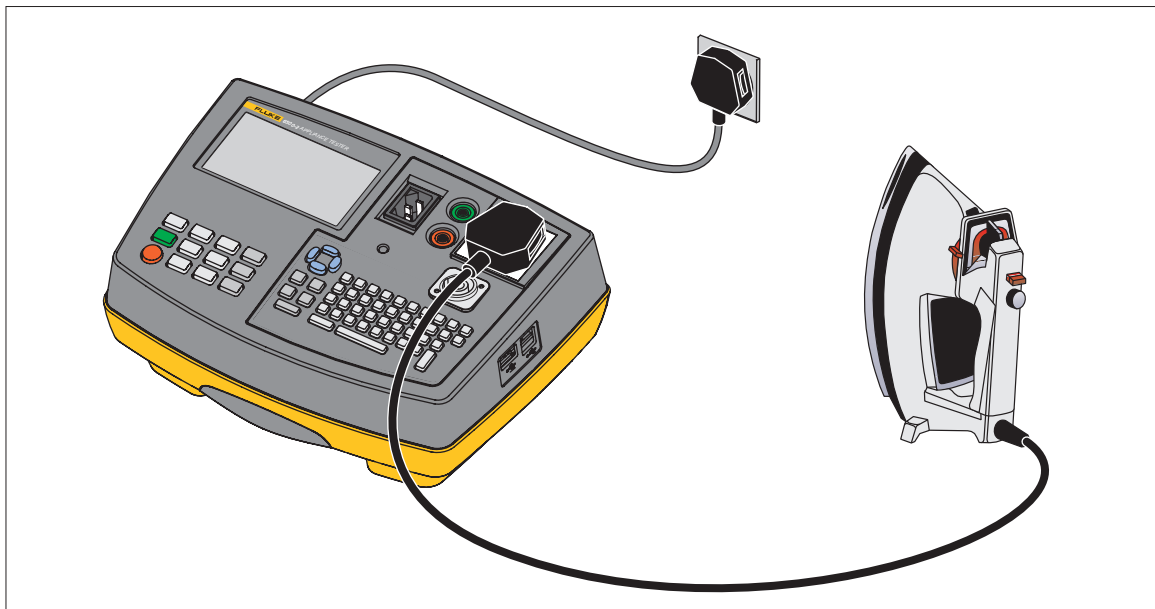
Abbildung 8. HF-Leckstrom-Testanschlüsse
